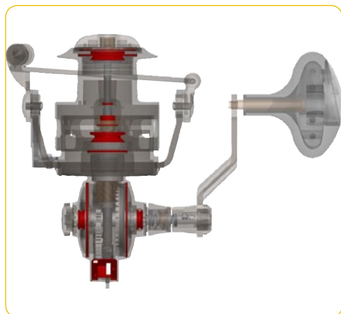
Die roten Markierungen zeigen die 13 versiegelten Stellen in der Rolle an.
